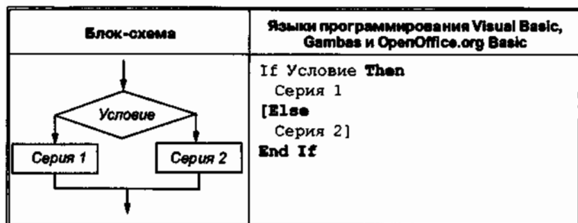
Рис. 4.3. Алгоритмическая структура «ветвление»
