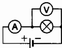
Рис. 5.6. Электрическая схема
