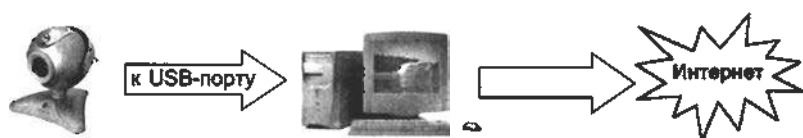
Рис. 1.27. Потоковое видео
