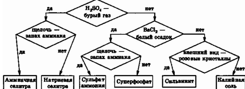
Рис. 5.17. Блок-схема экспертной системы «Распознавание удобрений»
