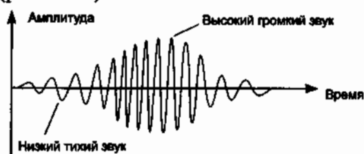
Рис. 1.23. Звуковая волна
