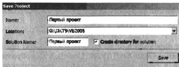
Рис. 4.1.3. Сохранение проекта
