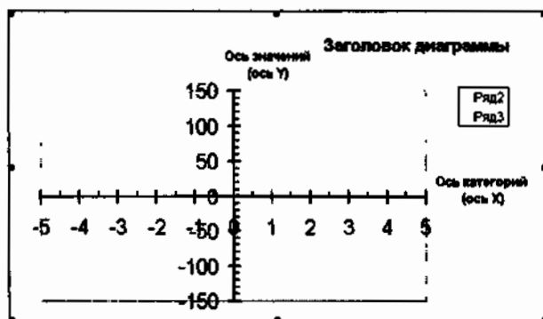
Рис. 3.8. Область диаграммы
