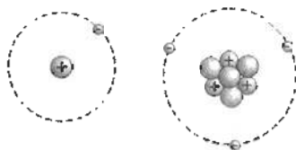
Рис. 5.4. Атом водорода и атом лития
